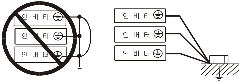
그림 5-2 AI-DS 접지 방법
