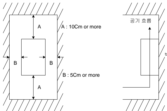
그림 5-1 AI-DS 설치 지침
